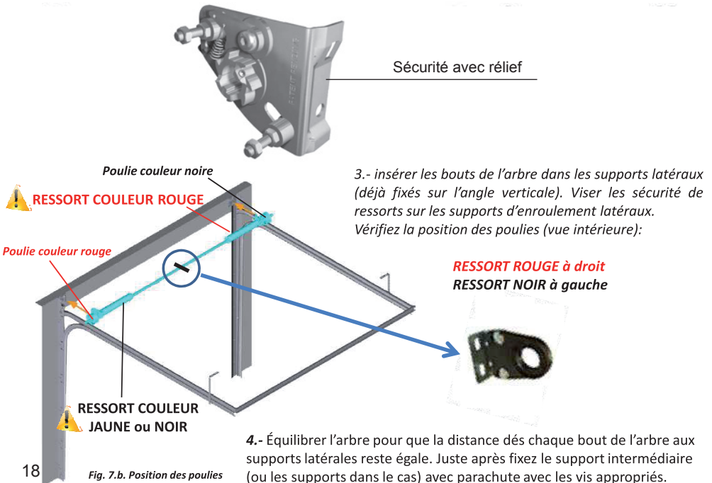
Fig. 7.b. Position des poulies
