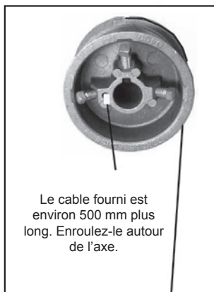
Fig.19 Réglage du câble d'acier tressé dans le butoir du tambour
