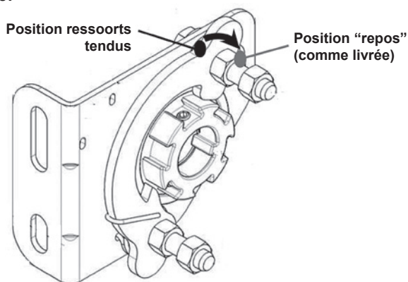
Fig. 21: la position du boulon supérieur varie quand les ressorts sont tendus.
