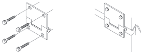
Fig.10 Installation des supports de galet latéraux et les charnières intermédiaires
