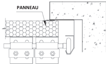
Fig.15 Réglage du support de galet DOUBLE
