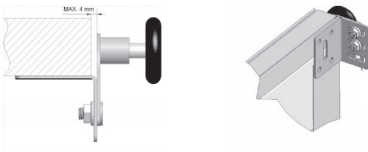
Fig.13 Support de galet supérieur pour le linteau réduit (D160)
