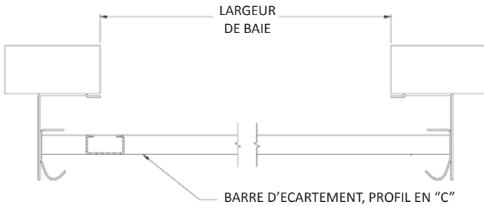
Fig. 5 emboîtement de la barre d'écartement
