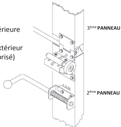
Fig.16 Placement du verrou manuel intérieur
