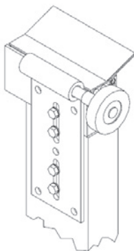
Fig.12 Support de galet supérieur pour le linteau réduit (D200)
