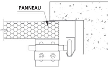
Fig.14 Réglage du support de galet SIMPLE
