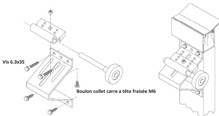
Fig.11 Support de galet supérieur pour des linteaux standards (D300, D350 & D420)
